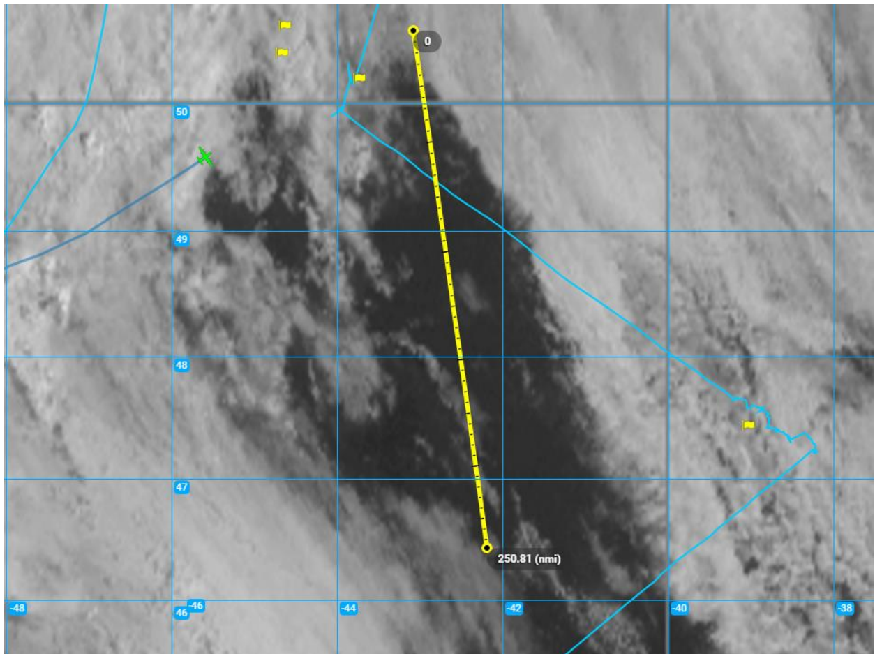
1220Z_InTheBoxTowardS3
