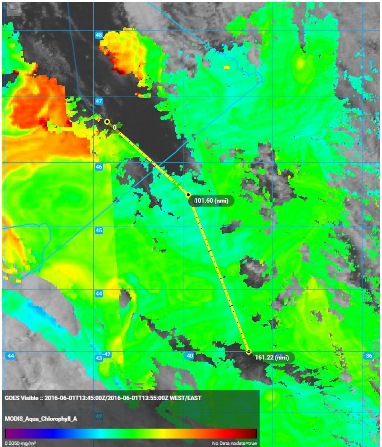
1405Z_SouthboundHighAltRunOnTheKinkWithMay24thChlorophyll
