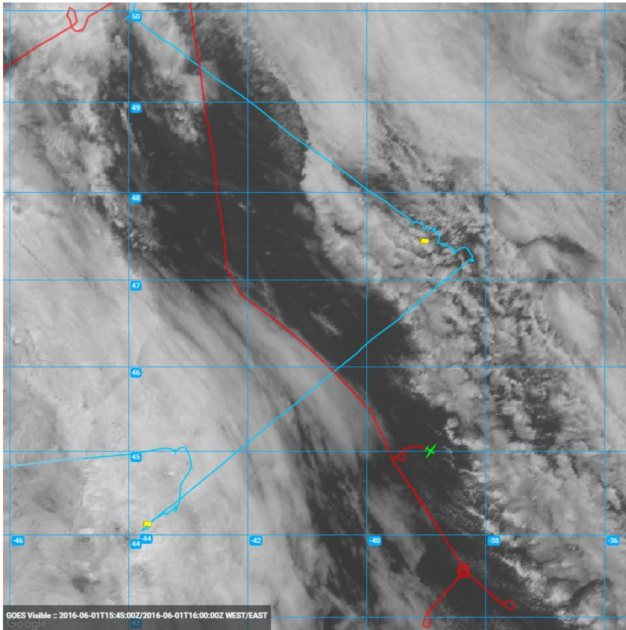
1610Z_SpiralUpDuringLowAltLeg
