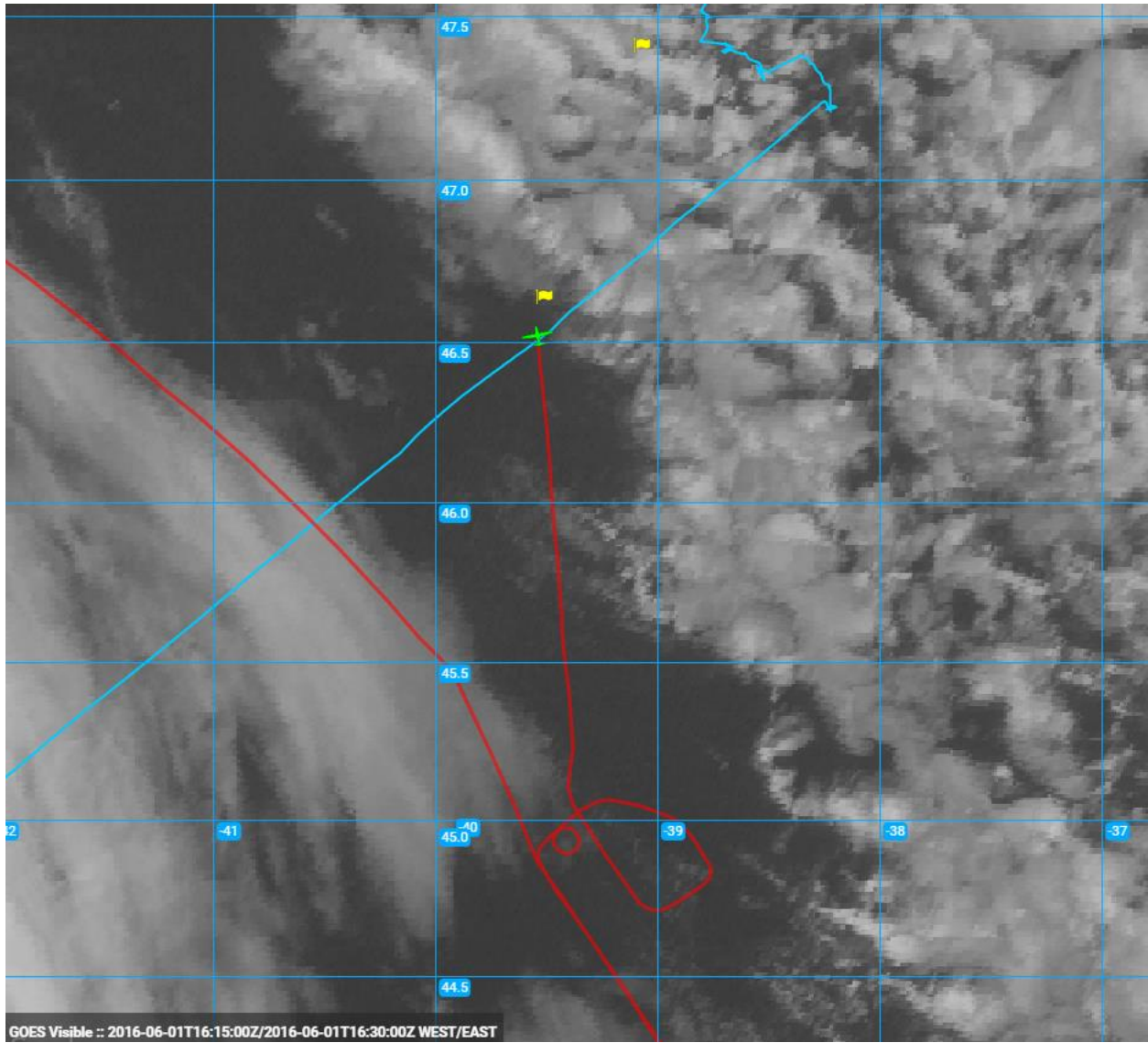
1640Z_FloatOverflight
